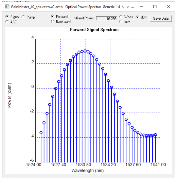
Рис. 2а. АЧХ EDFA без GFF и АТТ2
