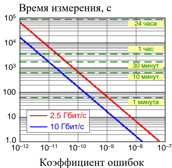
Рис. 1. Зависимость времени измерения от ожидаемого BER
