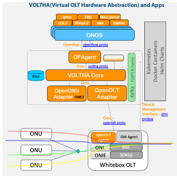
Рис. 3. Структура VOLTHA
