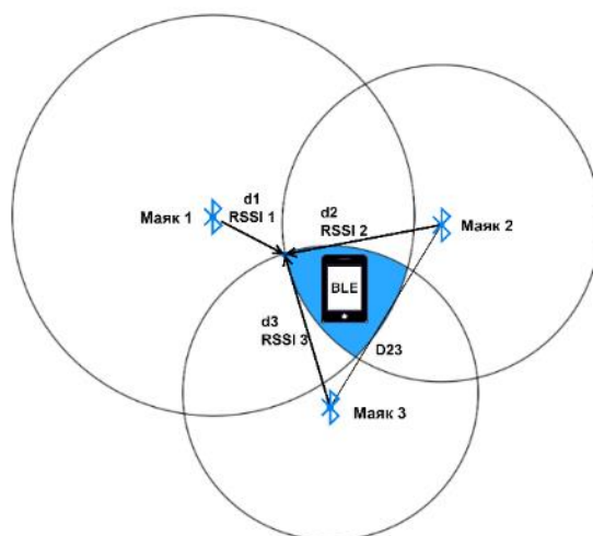
Рис. 1. Трилатерация
