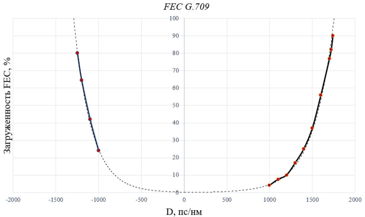
Рис. 3. График зависимости загрузки FEC G.709 от величины дисперсии
