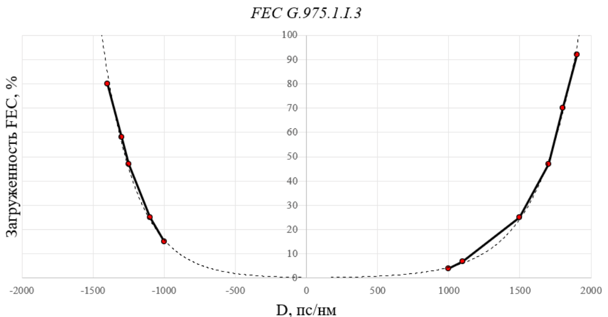
Рис. 4. График зависимости загрузки G975.1.1.3 от величины дисперсии
